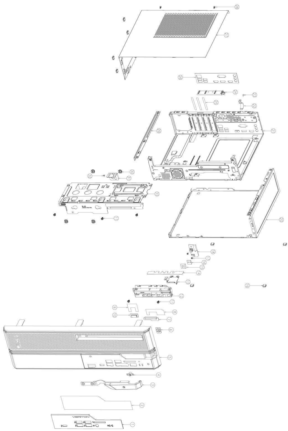
圖 1 系統分解圖
