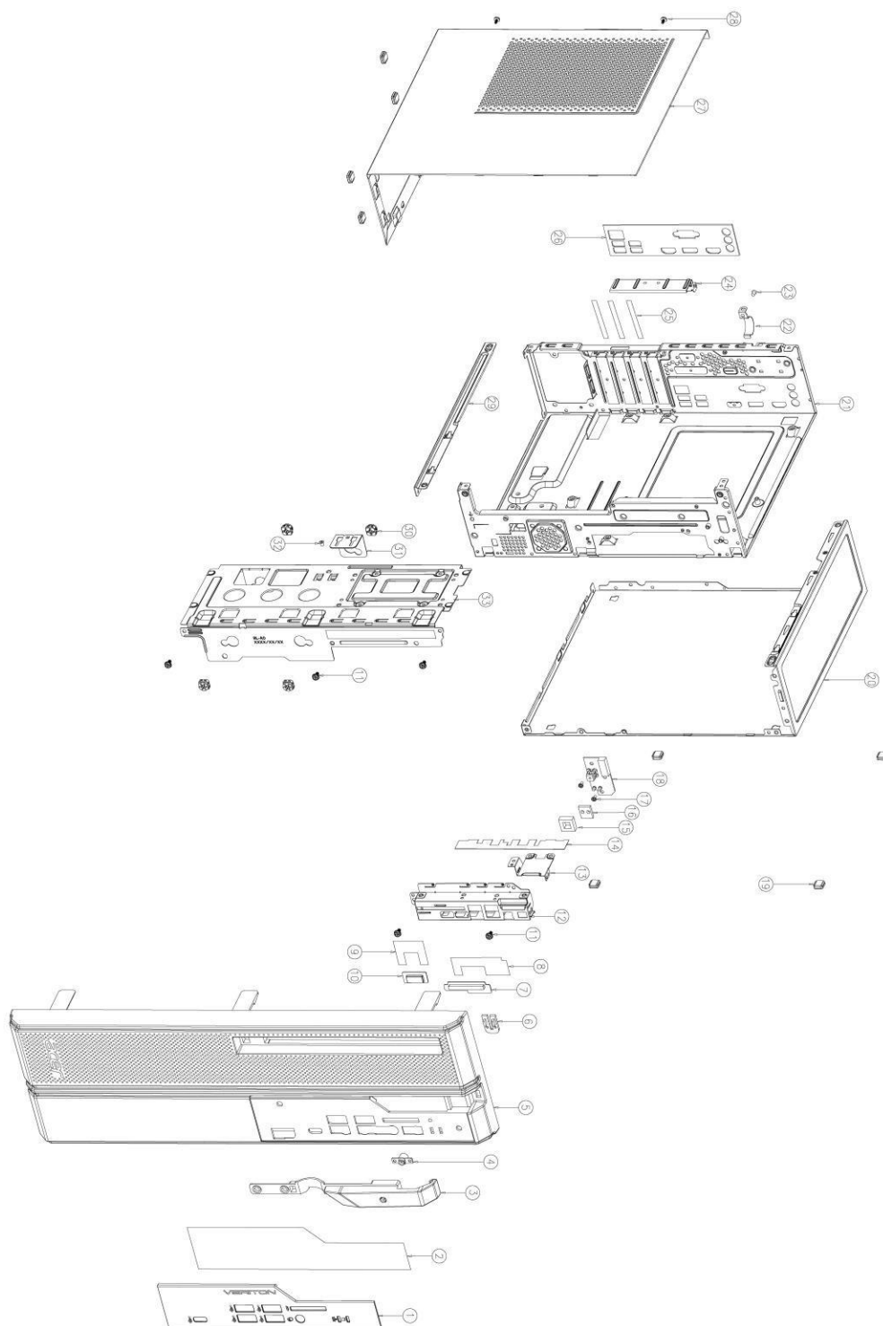
Rysunek 1 Schemat rozłożony systemu
